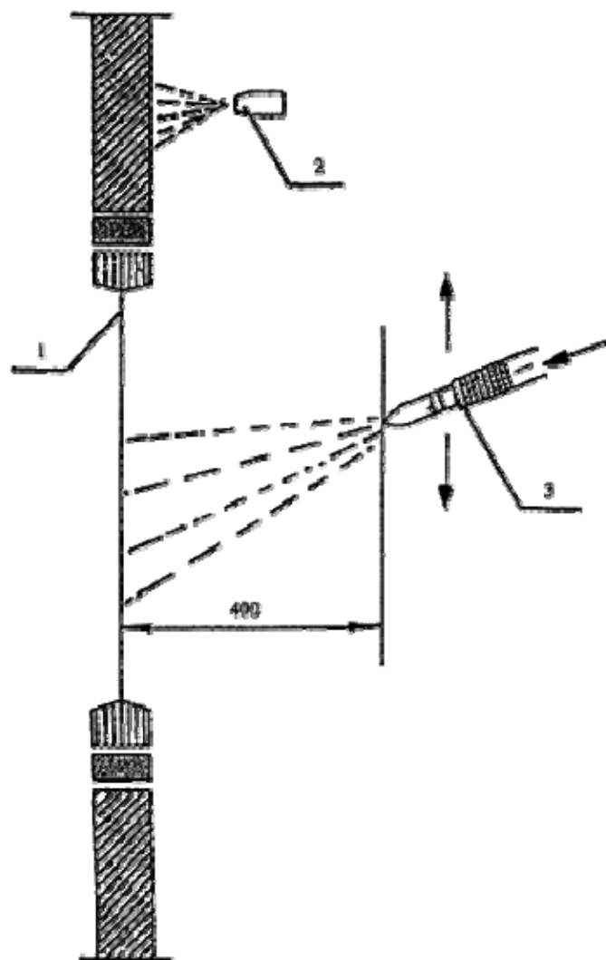
1 - образец; 2 - форсунка верхнего неподвижного ряда; 3 - подвижная форсунка
