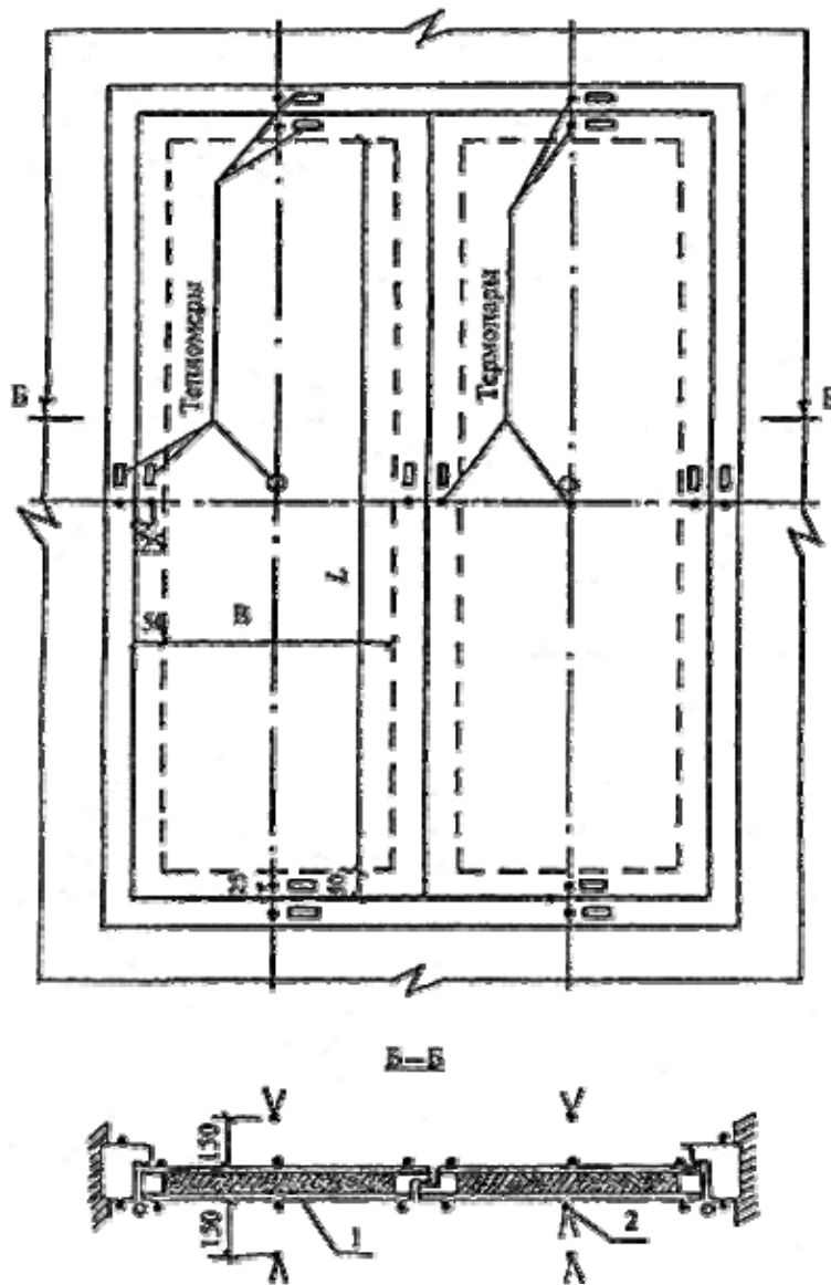
1 - испытываемый образец; 2 - рабочий спай термопары
