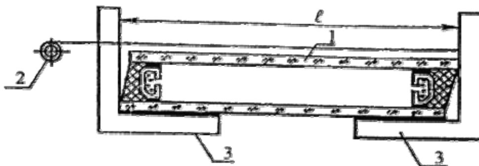
1 - стеклопакет; 2 - рулетка; 3 - угольник; i - контролируемый размер
