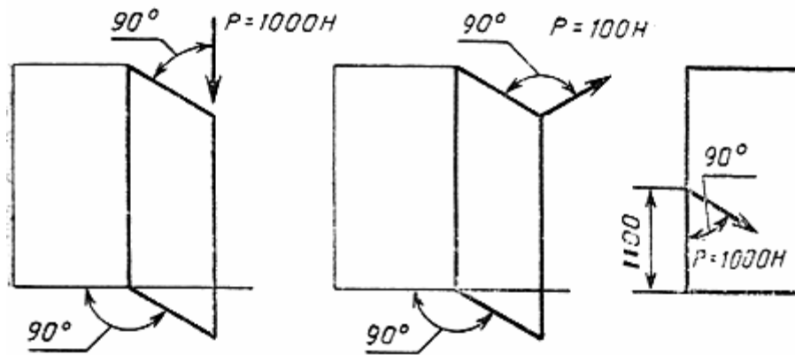
Дверь с распашными и качающимися полотнами
