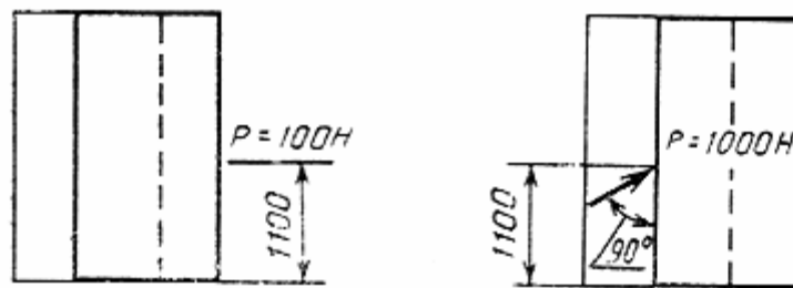
Дверь с раздвижными полотнами
