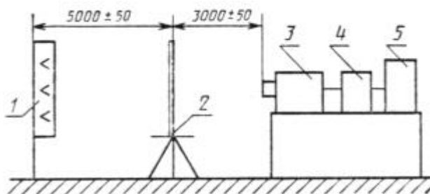
Схема установки для определения оптических искажений стекла
